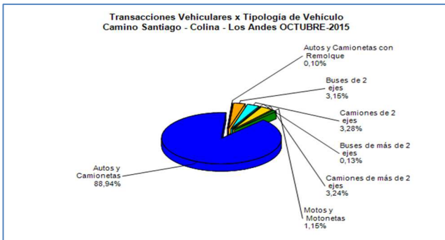
Gráfico 2: Distribución de Flujos de Octubre 2015, por categoría de vehículo Fuente: Reporte SICE 29
